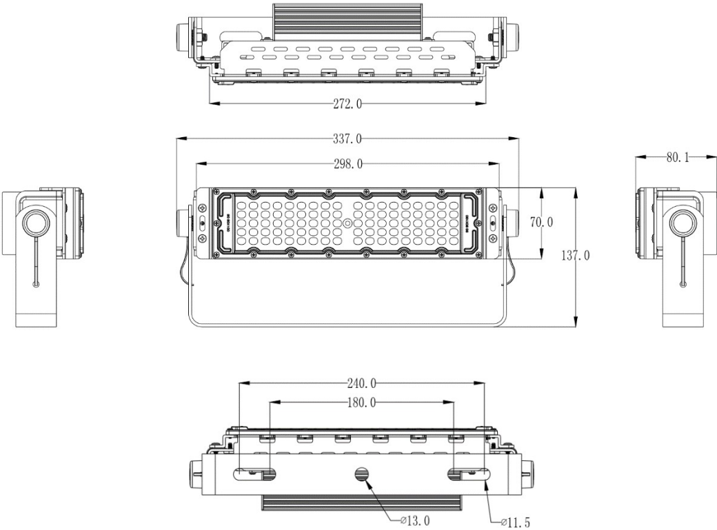
ZTS-100 外形图
