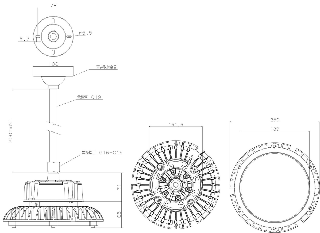
天井直付けタイプ外形図
