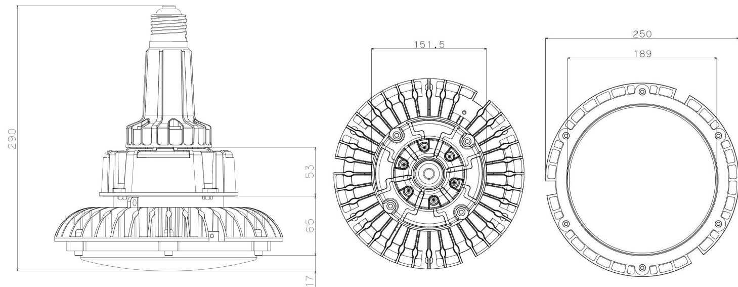
拡散タイプ外形図 (E39 口金)
