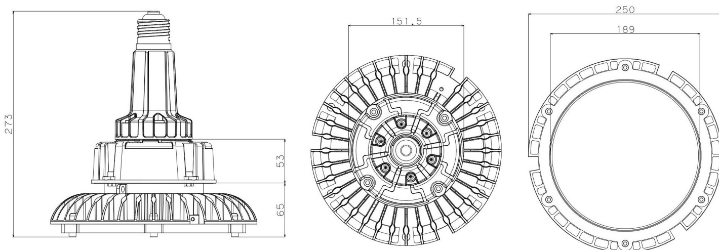
標準タイプ外形図 (E39 口金)
